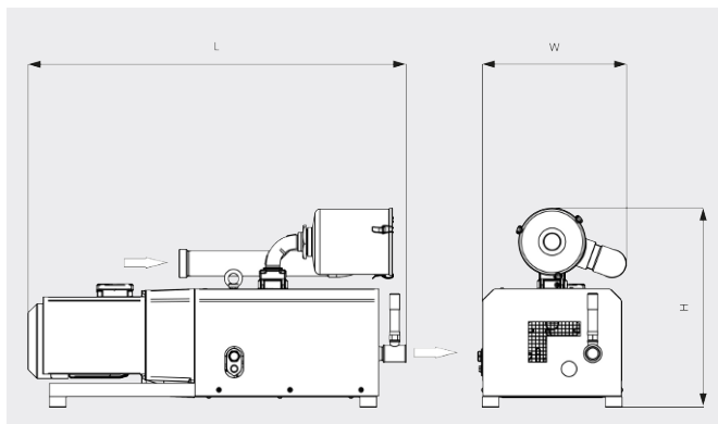
寸法図
