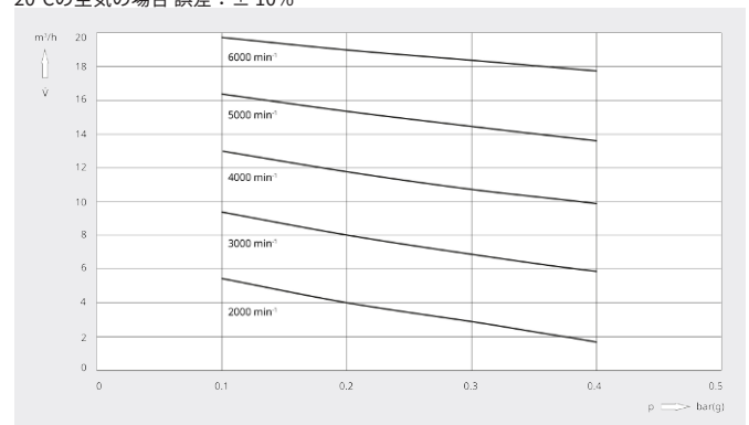
排気速度 20°Cの空気の場合 誤差：± 10%
