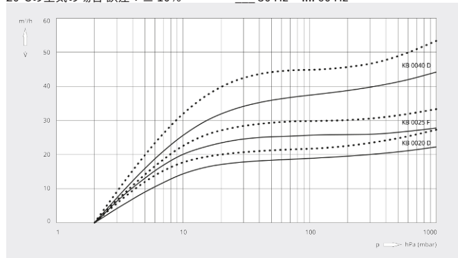
排気速度
