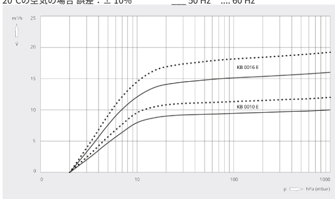
排気速度
