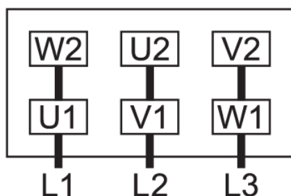
スター接続（高電圧）：
