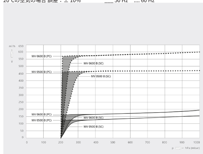
排気速度
