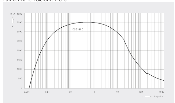
Saugvermögen Luft bei 20 °C. Toleranz: ±10 %
