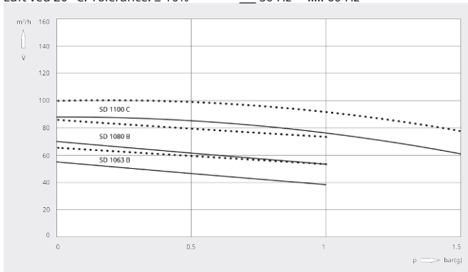
Volumenflow
