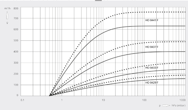
Pumpehastighed
