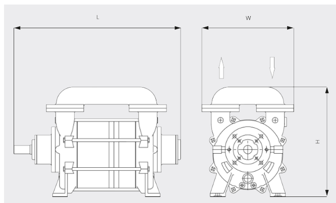
Måltegning
