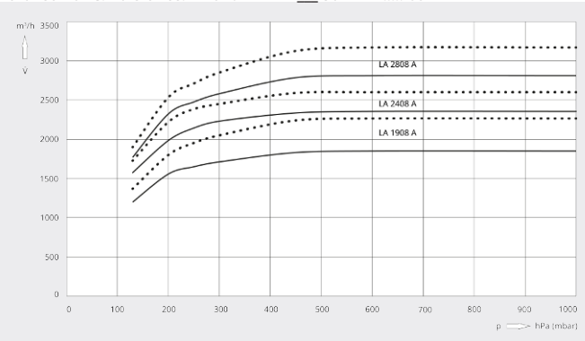
Pumpehastighed
