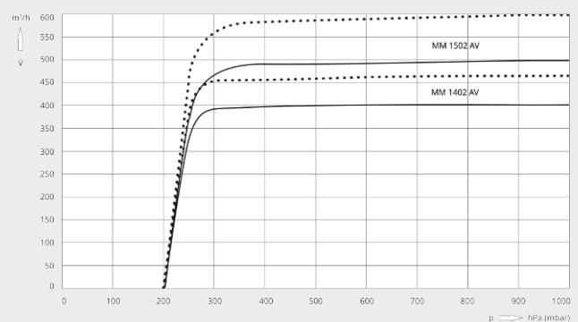
Pumpehastighed
