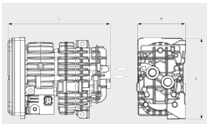
Måltegning
