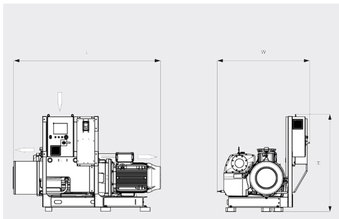
Måltegning
