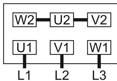
Stjerneforbindelse (højspænding):
