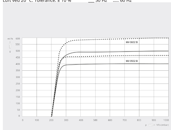
Pumpehastighed
