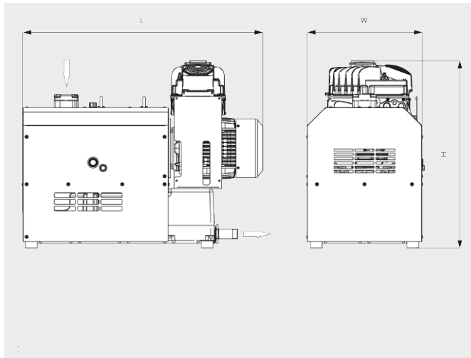
Måltegning
