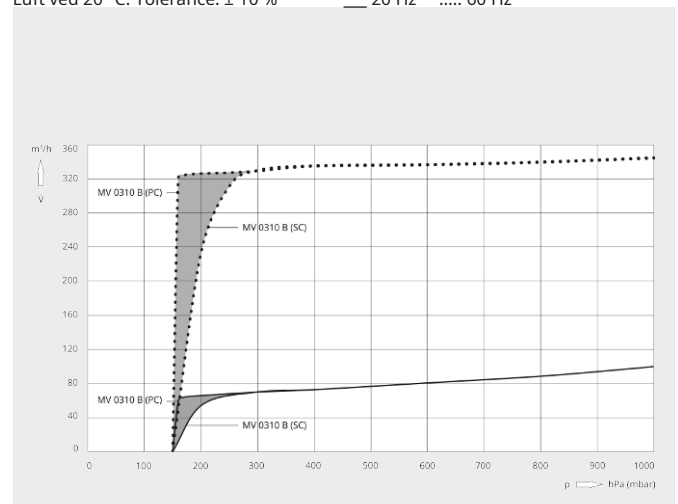
Pumpehastighed
