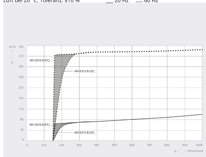
Saugvermögen
