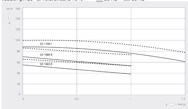
Objemový průtok
