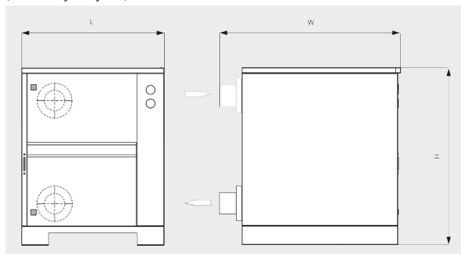
Rozměrový výkres (s akustickým krytem)
