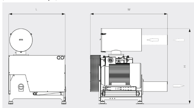
Rozměrový výkres (bez akustického krytu)
