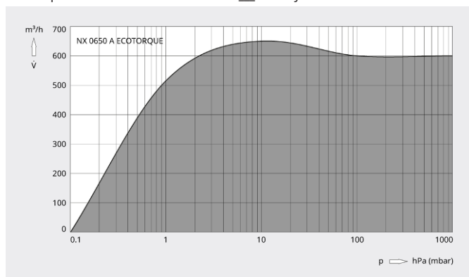
Rychlost čerpání
