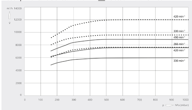
Rychlost čerpání
