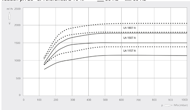
Rychlost čerpání
