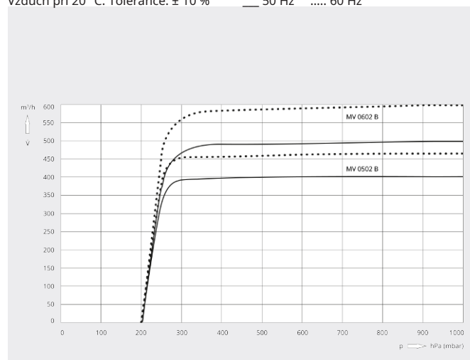
Rychlost čerpání
