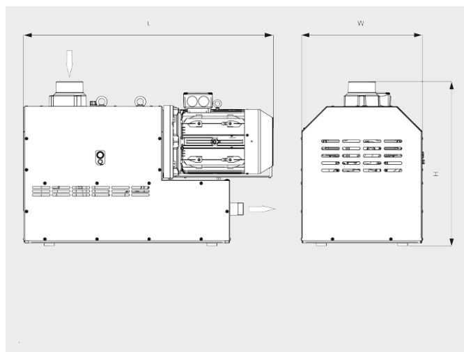
Rozměrový výkres
