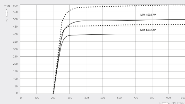
Rychlost čerpání
