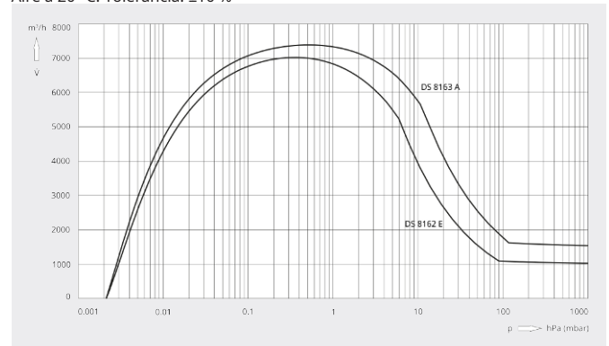
Caudal Aire a 20 °C. Tolerancia: ±10 %
