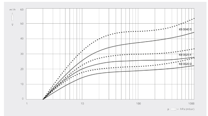
抽气速率
