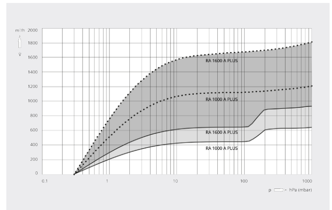
抽气速率
