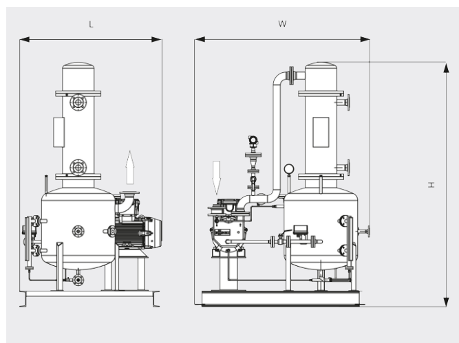
尺寸图
