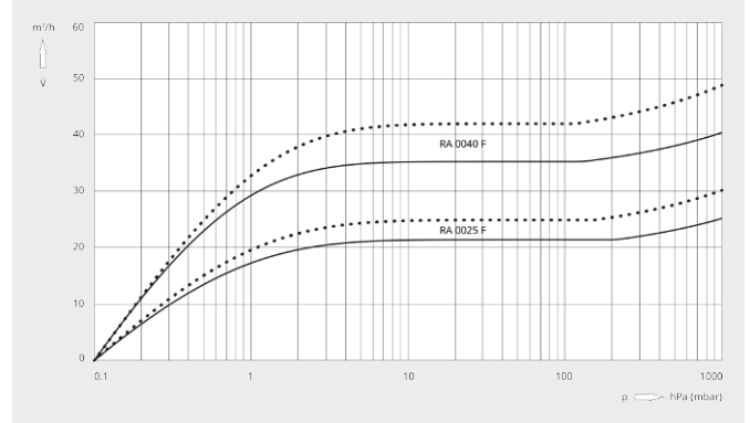
抽速
