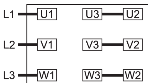
双星形连接，多电压电机，含 12 针（低电压）：
