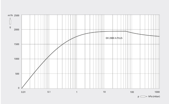
抽气速率 空气温度为 20 °C 时，公差：± 10%
