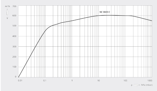
抽气速率 空气温度为 20 °C 时，公差：± 10%
