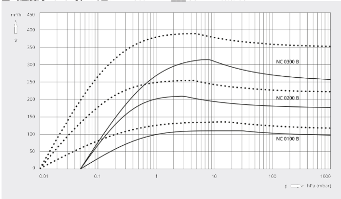
抽气速率 空气温度为 20 °C 时, 公差: \pm 10\% — 50 Hz ..... 60 Hz
