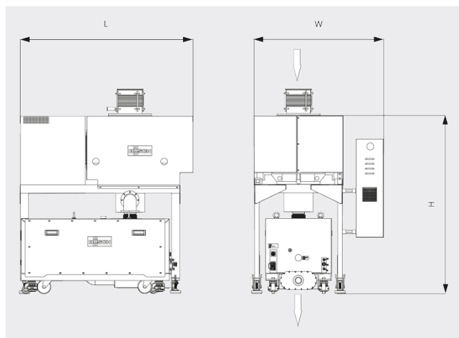
尺寸图
