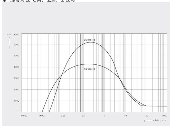
抽气速率
