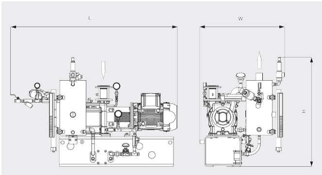
尺寸图
