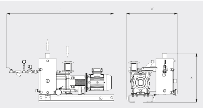
尺寸图
