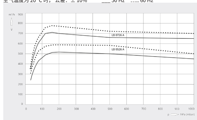
抽气速率
