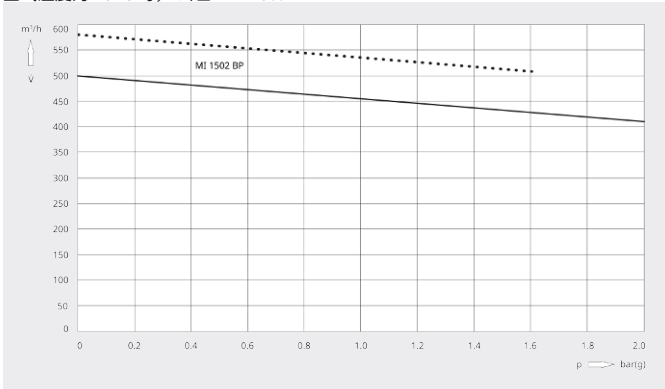
抽气速率 空气温度为 20 °C 时，公差：± 10%
