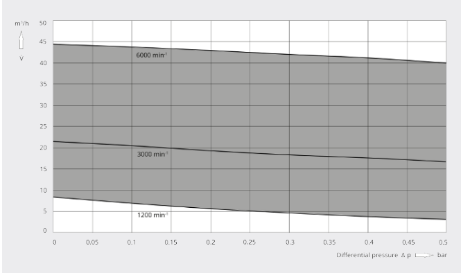
体积流量（进气口） 空气温度为 20 °C 时 公差：± 10%
