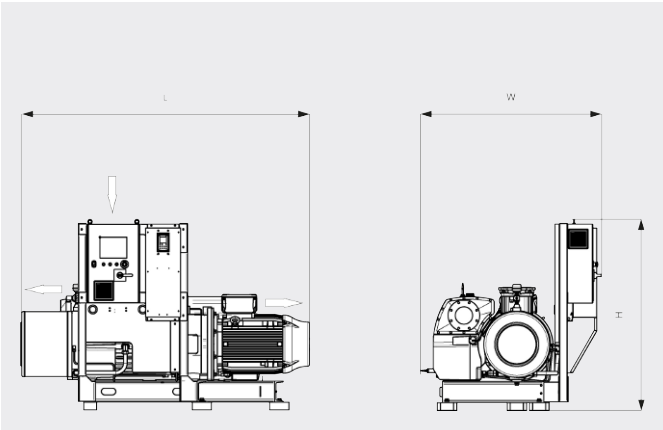
尺寸图
