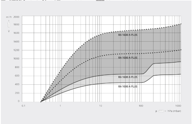
抽气速率
