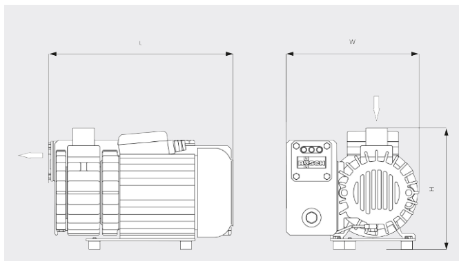
尺寸图
