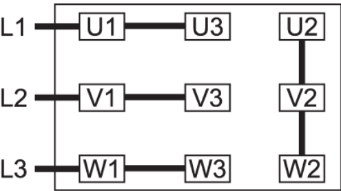
星形连接，多电压电机，含 9 针（高电压）：
