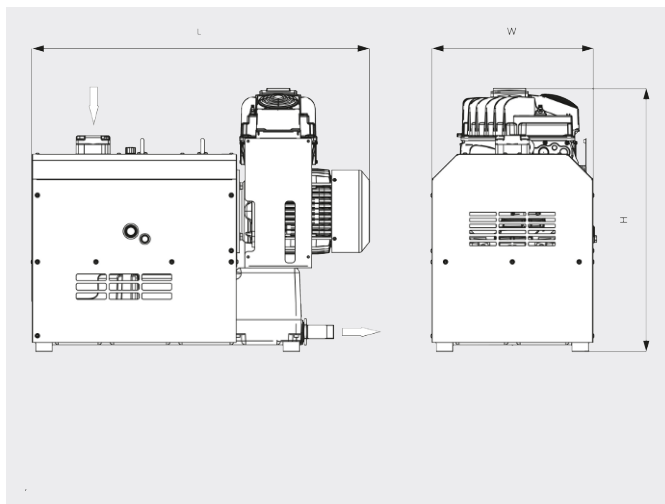
尺寸图
