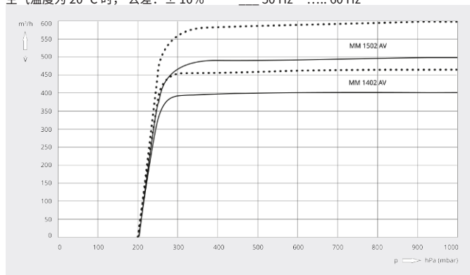
抽气速率
