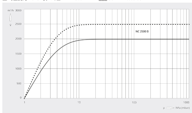
抽气速率
