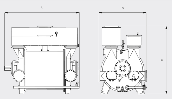
尺寸图
