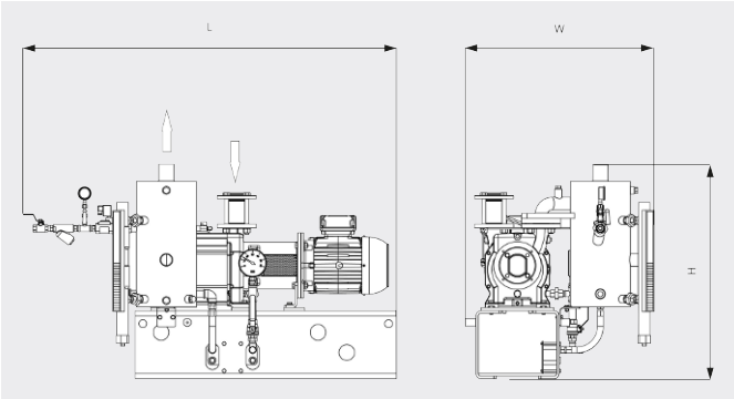
尺寸图
