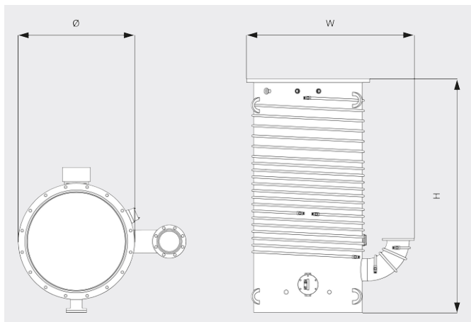
Dibujo dimensional
