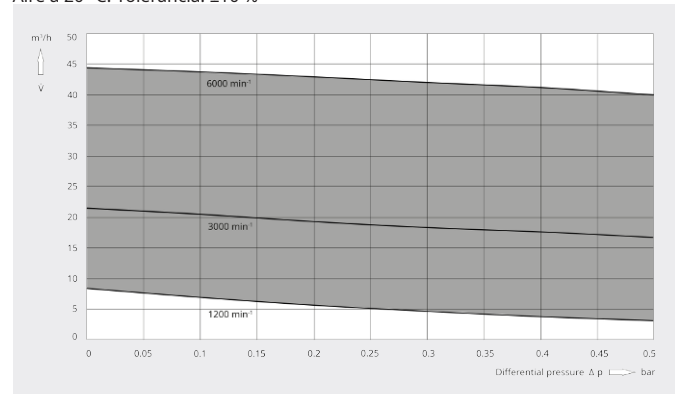
Caudal (en la entrada) Aire a 20 °C. Tolerancia: \pm 10\%
